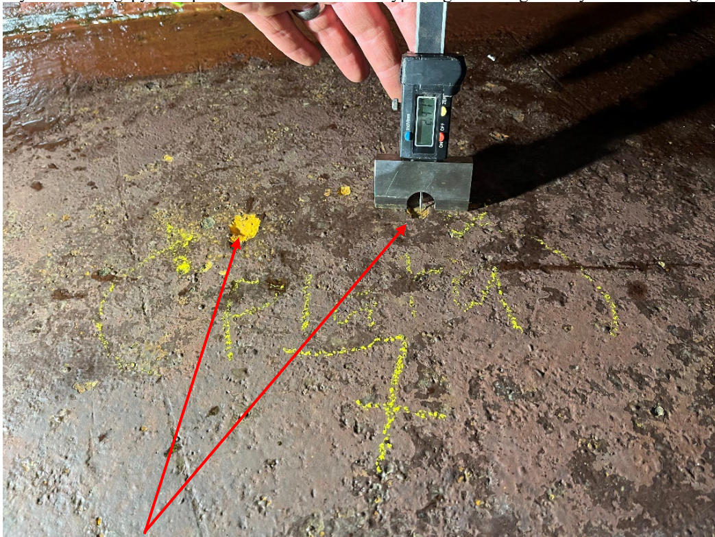
Mynd 10. Tæringapyttir á plötu 7 sem ná 2,7 og 2.4 mm að dýpt. Lagað að viðgerðarteymi olíudreifingar.
