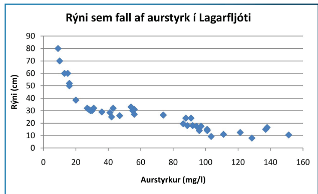
Mynd 7. Rýni sem fall af aurstyrk. Samband aurstyrks og rýnis við aurstyrk undir 15 mg/l er byggt á mælingum í Þórisvatni og Hvítárvatni en við hærri aurstyrk í Lagarfljóti (mynd frá Hákon Aðalsteinssyni, 2010).
