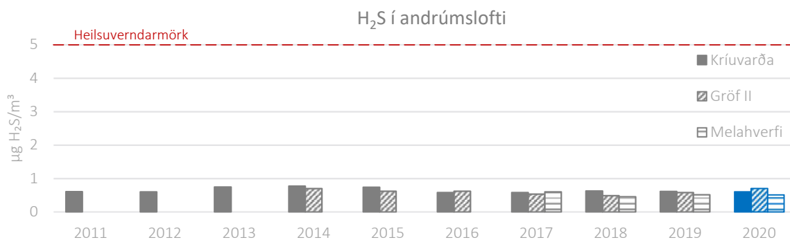
MYND 4.7 Meðalstyrkur \text{H}_2\text{S} á Kríuvörðu, Gröf II og Melahverfi.
