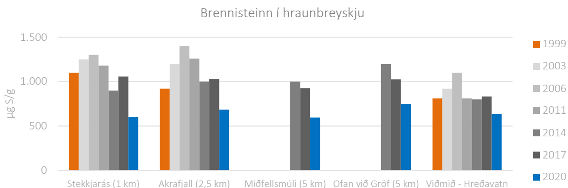
MYND 7.5 Styrkur brennisteins í snepaskóf ( Parmelia saxatilis ) og í hraunbreyskju ( Stereocaulon vesuvianum ) frá því að mælingar hófust.
