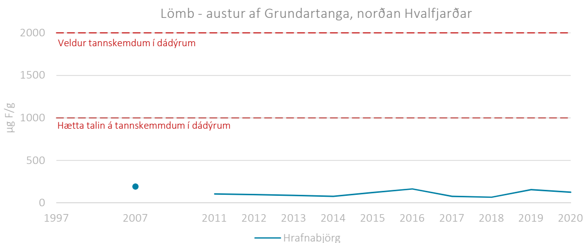
MYND G.1 Meðalstyrkur flúors í kjálkabeinum lamba frá bæjum austur af iðnaðarsvæðinu.
