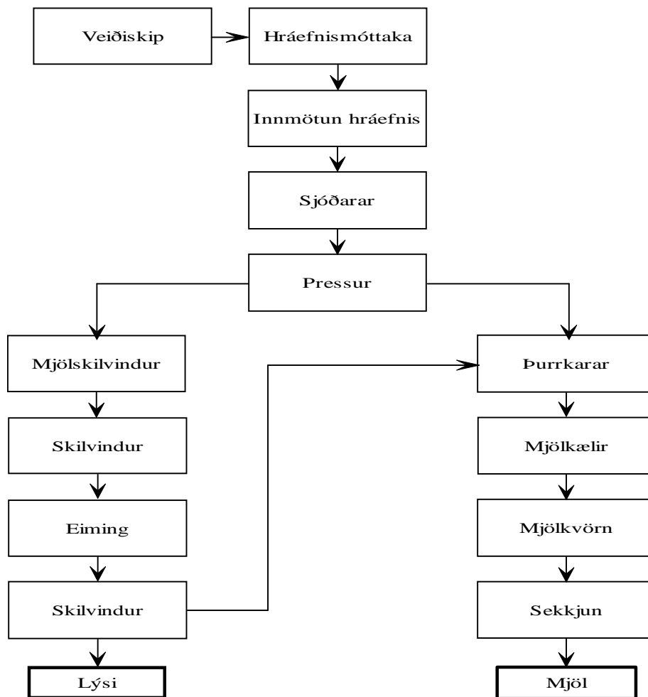
Mynd 2 Flæðirit verksmiðjunnar
