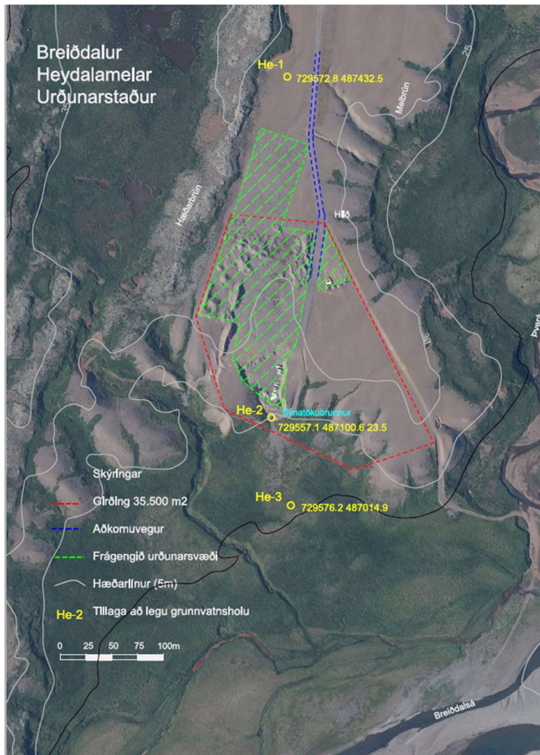
Mynd 1. Heydalemelar, urðunarstaður, staðsetning grunnvatnshola merkt inn.
