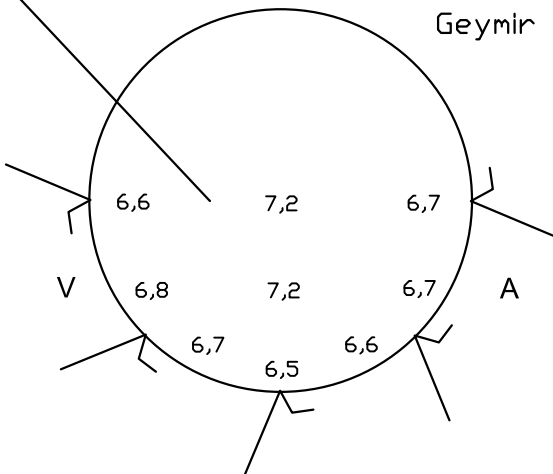
Staðsetning mælipunkta.
